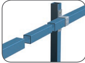
Kelepçe Bağlantı Detayı 1
