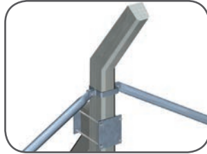
Boru Payanda ve Kelepçesi
