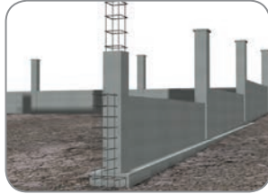
Betonarme Duvar 2
