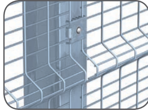
Metal Klips 2 (Yüksek Güvenlik Panellerinde)
